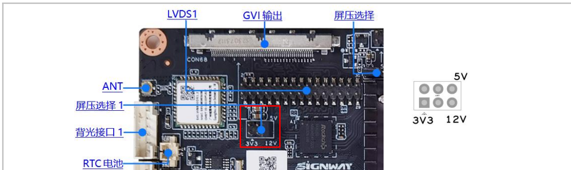
上图中用跳线帽来进行屏电源的选择 CON7 从左到右, 依次为: 3.3V / 5V / 12V
